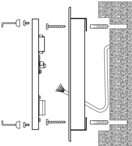
Montaż kasety w ramce podtynkowej
