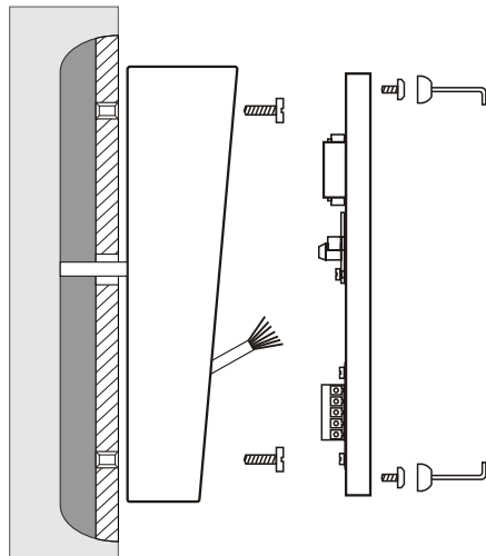
Montaż kasety w obudowie natynkowej
